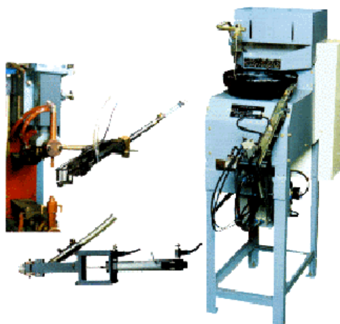
Bultmatare med vakuumbhållning av bulten, Även omagnetiska bultar matas (ex. rostfritt, aluminium). God åtkomlighet i trånga detaljer.
