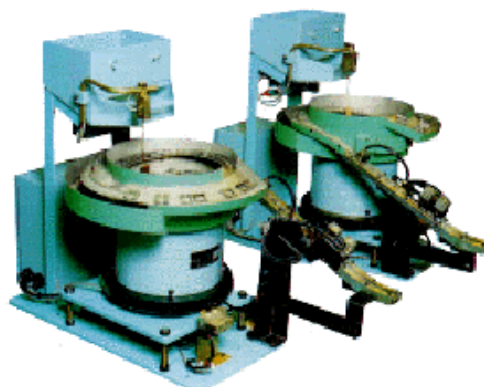
Komponentmatare, specialdesignad Detaljmatare för alla applikationer.
